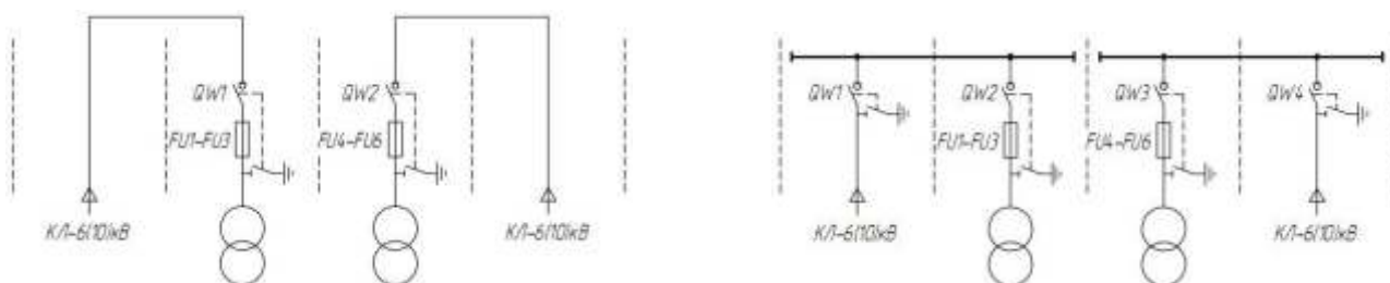
ТКв(к) 250 -1000кВА (с секционированием)
