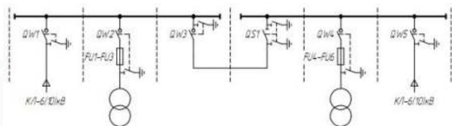
ТКв(к) 250 -1000кВА (с секционированием)
