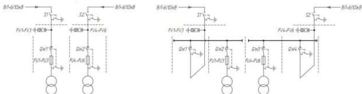
ТВв(к) 250 -1000кВА (с секционированием)
