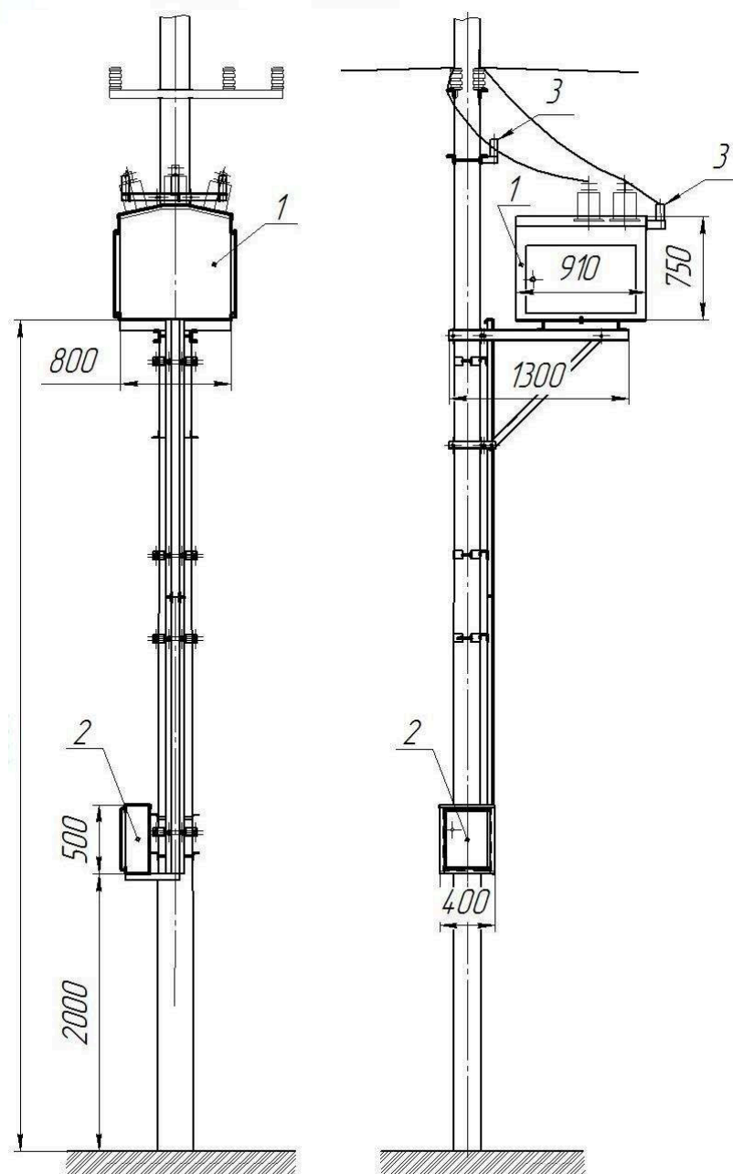
1 – Короб ПКУ; 2 – Ящик учета; 3 – ОПН
