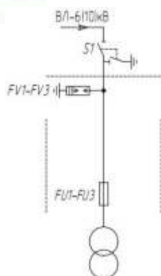
ТВв(к) 25 -400кВА (глухой ввод)
