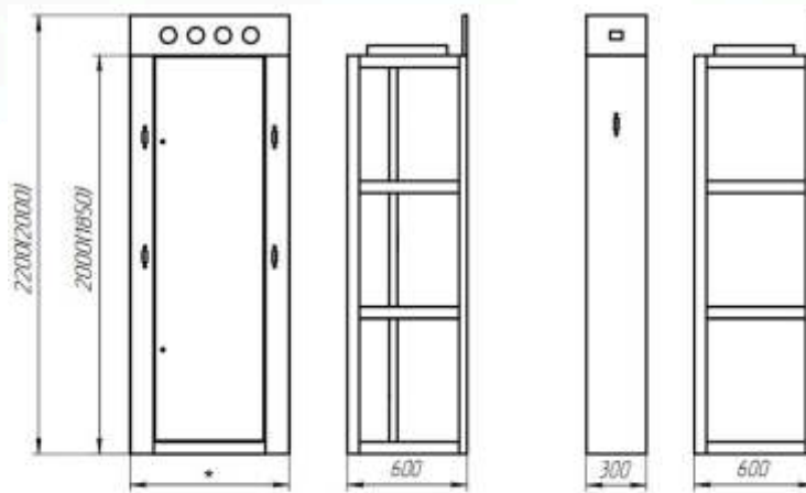
*Габаритные размеры ЩО70 зависят от типа ячейки
